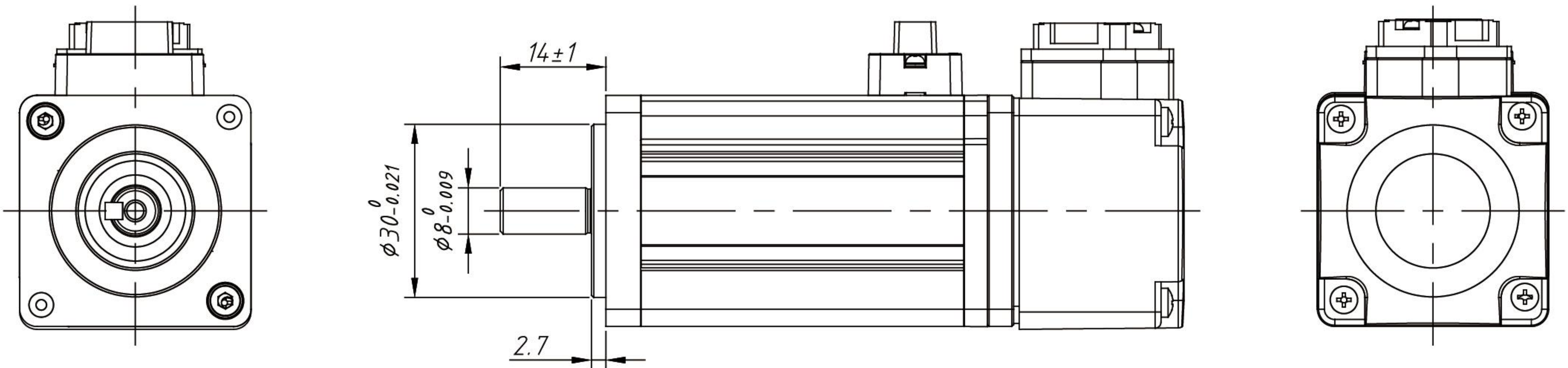
电机配合机械尺寸图 Mechanical Dimensions
