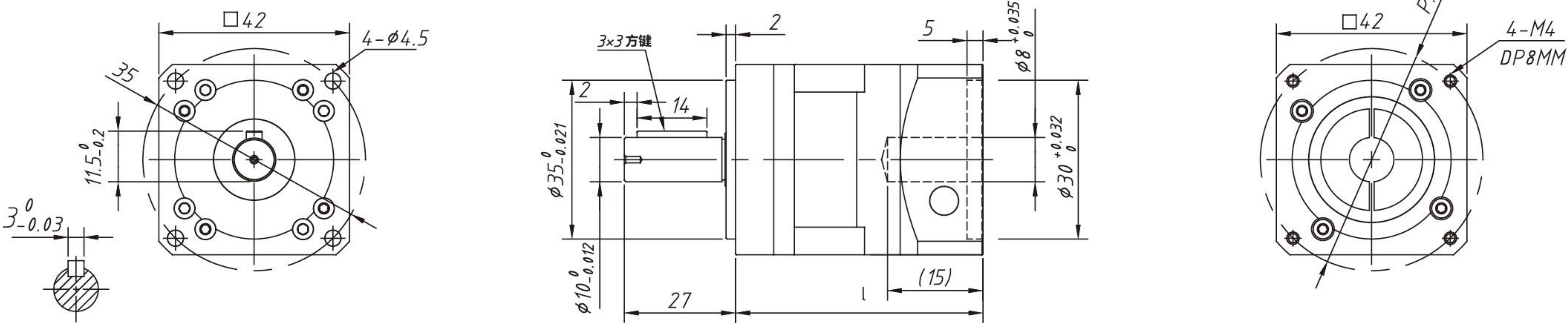
减速机机械尺寸图 Mechanical Dimensions 前方后方式
