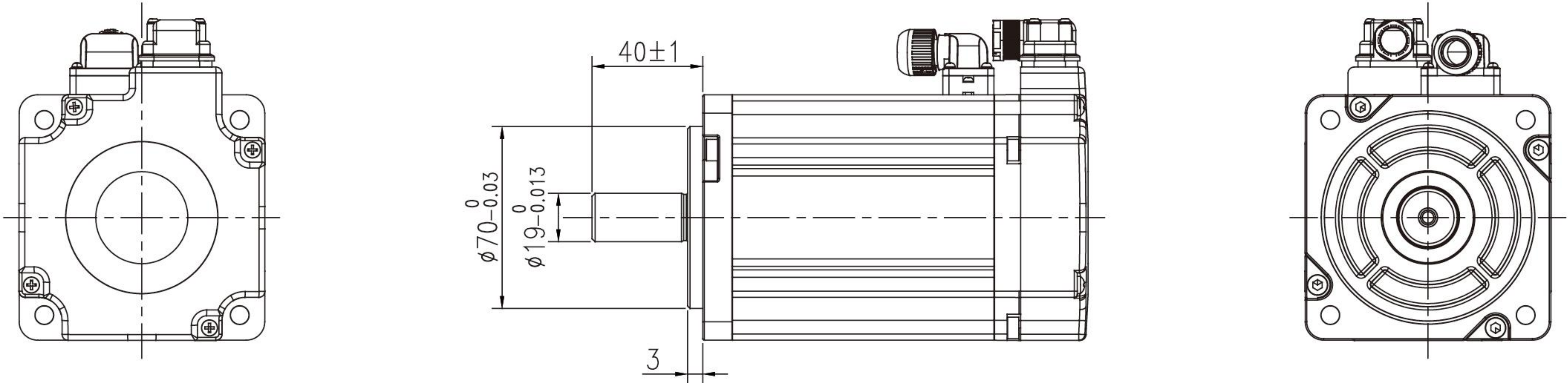
电机配合机械尺寸图 Mechanical Dimensions
